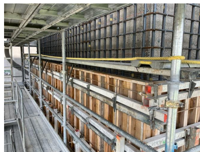
④琵琶川橋 左：型枠組立完了(3PB) 右：生コン打設状況(3PA・3PB)
