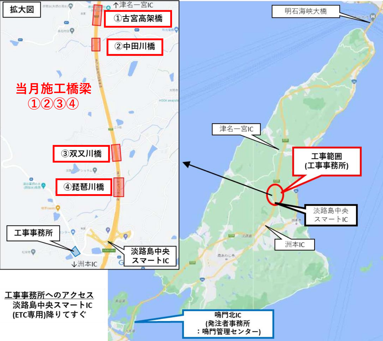
施工位置図
