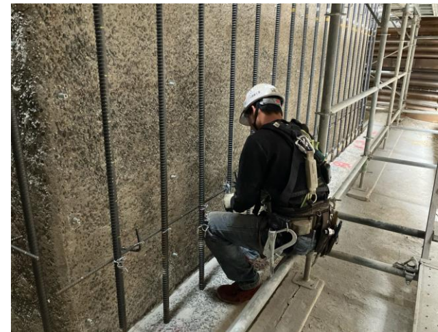
④琵琶川橋 左：既設躯体表面処理状況(5PA) 右：鉄筋組立状況(3PB)
