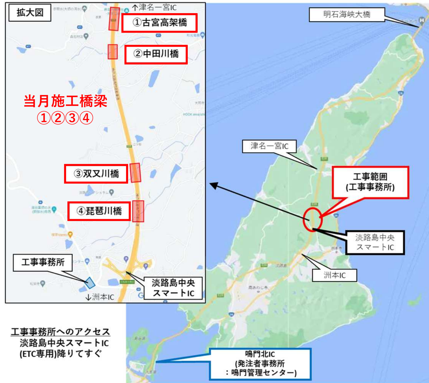
施工位置図
