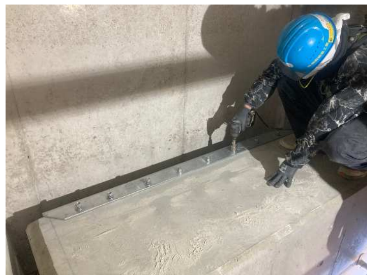
①古宮高架橋 左：緩衝ゴム設置状況(4PA) 右：鉄筋組立状況(5AA)
