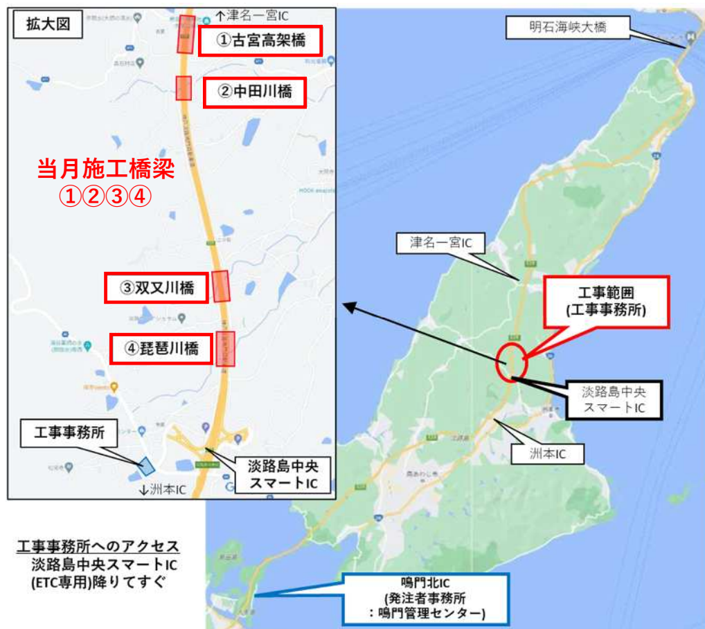
施工位置図
